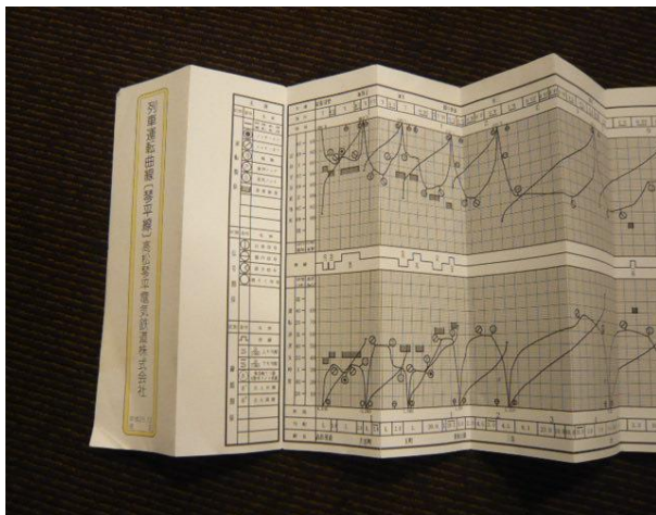
運転曲線
